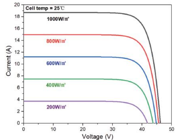
不同辐照度下I-V曲线(SP-G12/132H675W)
