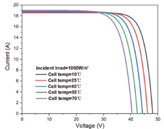
不同工作温度下I-V曲线(SP-G12/132H675W)
