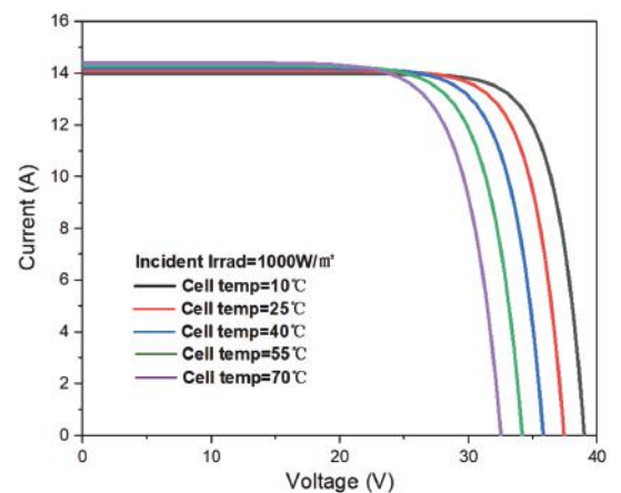
不同工作温度下I-V曲线(SP-M10/108H415W)
