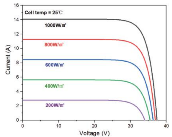
不同辐照度下I-V曲线(SP-M10/108H415W)
