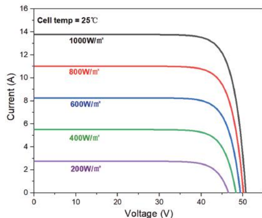
不同辐照度下I-V曲线(SP-M10/144H560W)
