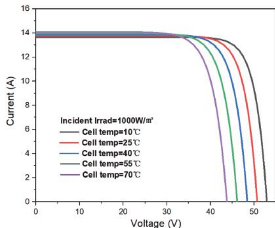
不同工作温度下I-V曲线(SP-M10/144H560W)
