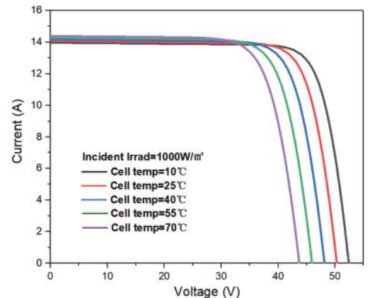
不同工作温度下I-V曲线(SP-M10/144H555W)
