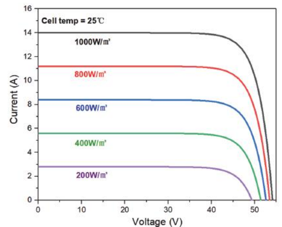
不同辐照度下I-V曲线(SP-M10/156H600W)
