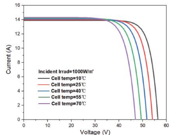
不同工作温度下I-V曲线(SP-M10/156H600W)
