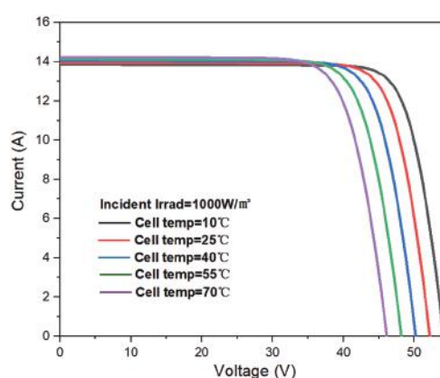
不同工作温度下I-V曲线(SP-N16/144HG580W)
